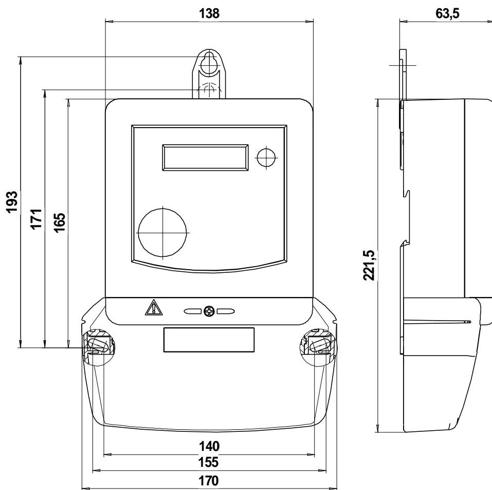
Внешний вид счетчиков НЕВА МТ31Х
