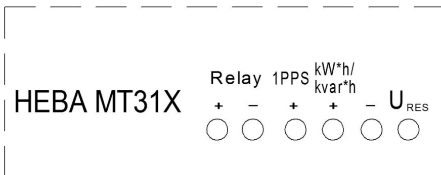
Схема подключения испытательных выходов счетчиков HEBA MT315 с промежуточным реле управления нагрузкой
