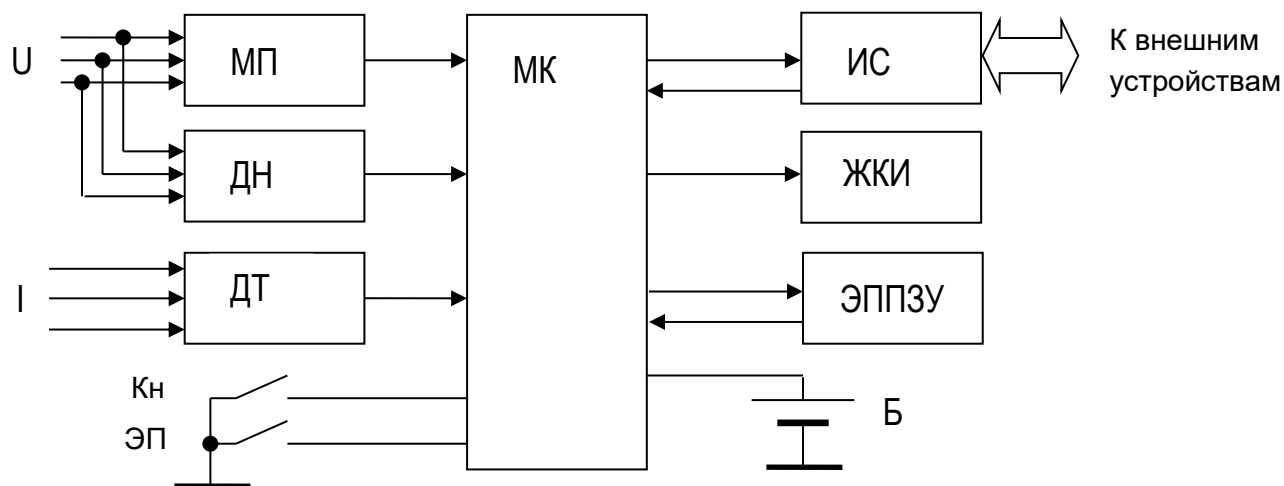
Рисунок 1 Функциональная схема счётчика.
