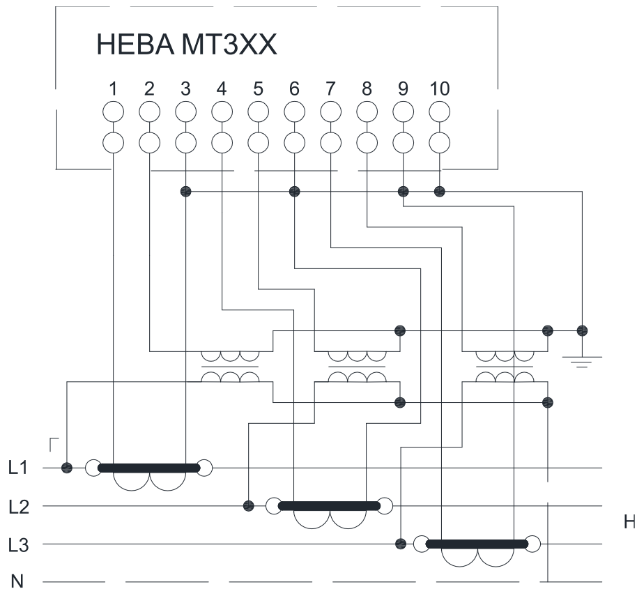
Схема включения счетчиков HEBA MT3XX через трансформаторы тока и трансформаторы напряжения в трёх- и четырёхпроводную сеть. Подключение к трёхпроводной сети осуществляется без подключения нулевого проводника.
