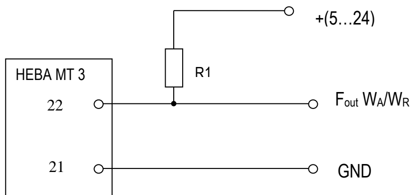
Рисунок 2.1 Подключение испытательных выходов счетчиков НЕВА МТ3
